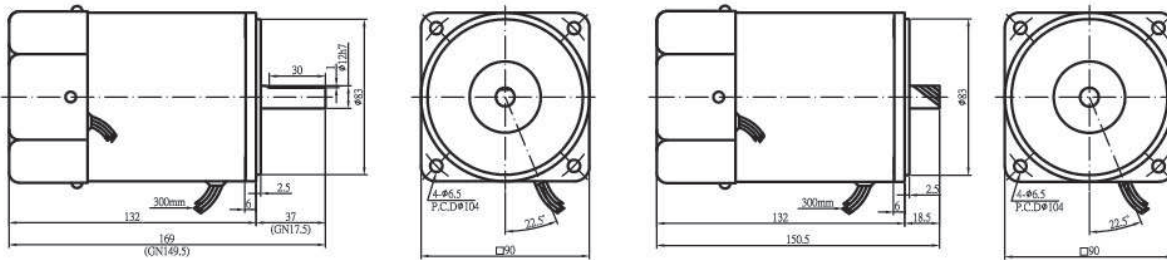
60W/60W-GX外型圖
